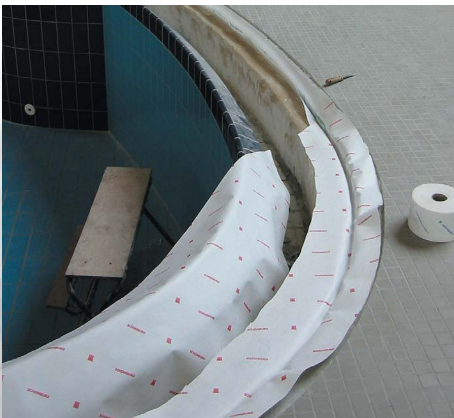
Повреждения посредством некачественной гидроизоляции деформационного шва
